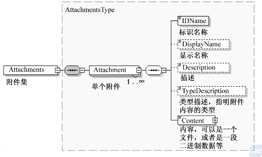
图 4 附件集示意图
