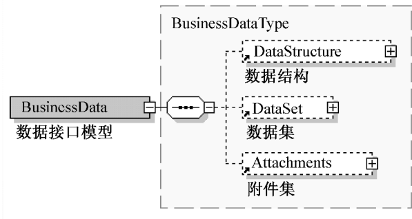
图 1 数据接口模型示意图
