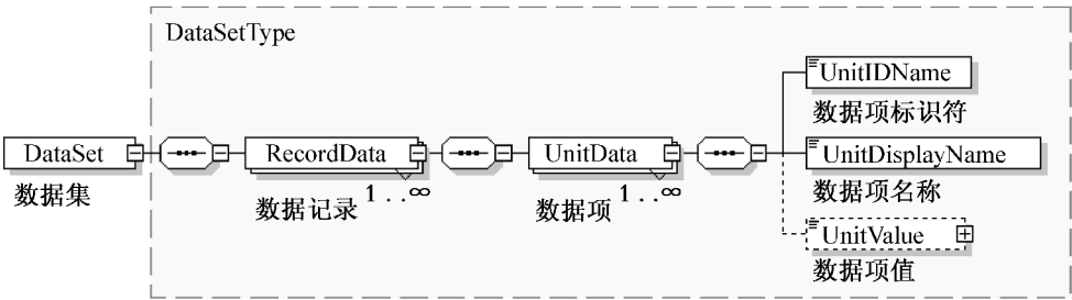
图 3 数据集示意图
