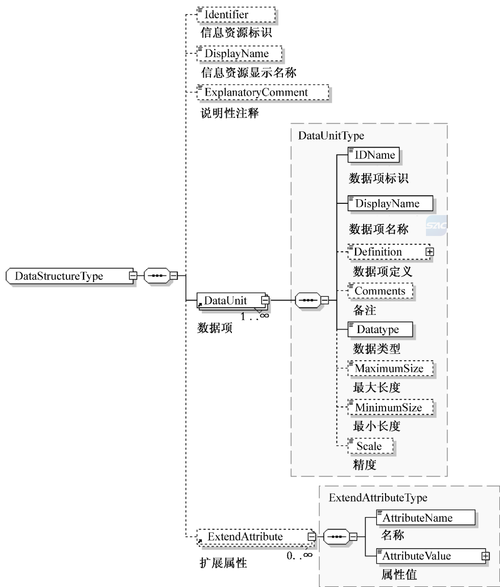
图 2 数据结构示意图
